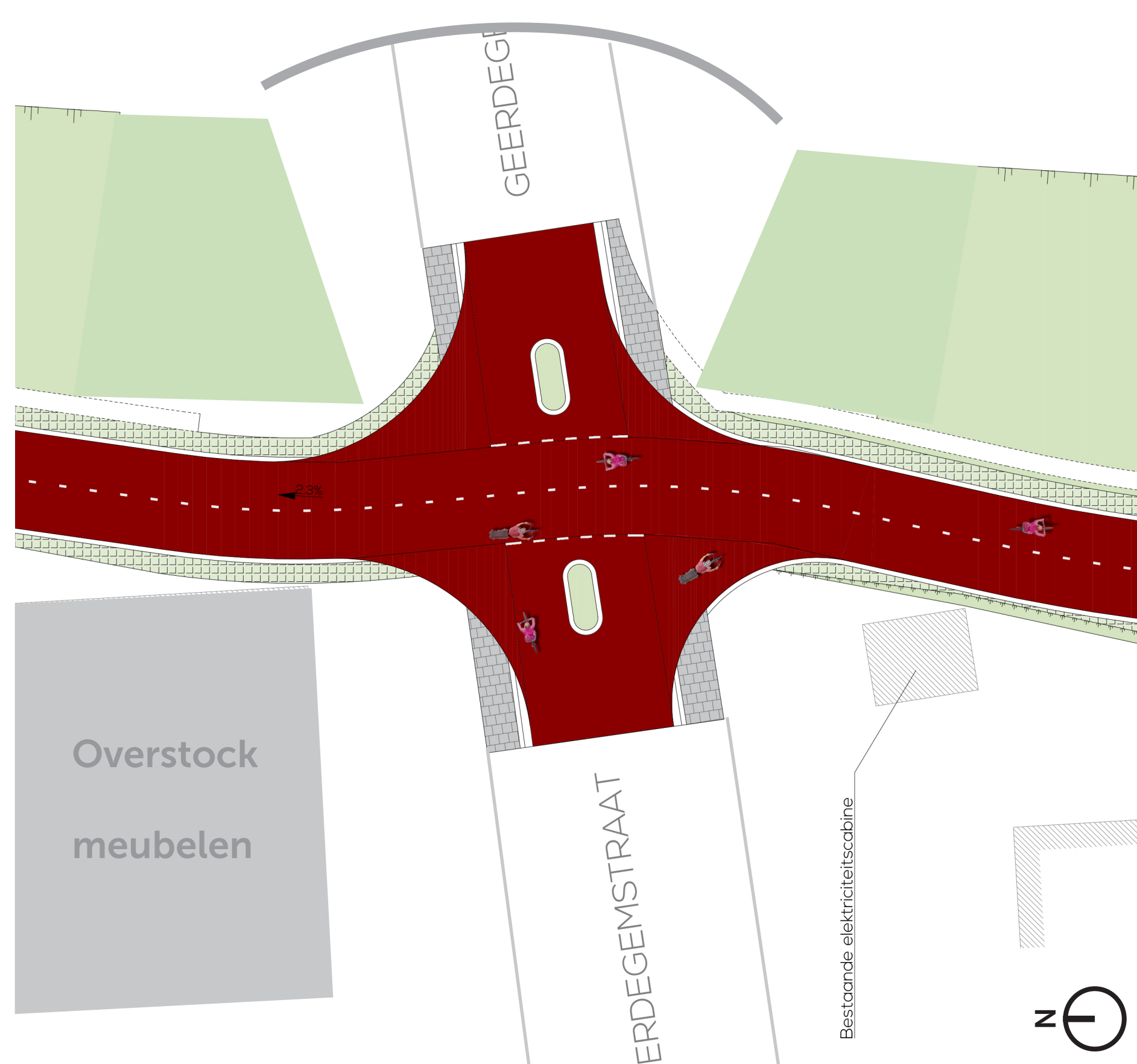
Grondplan kruising
