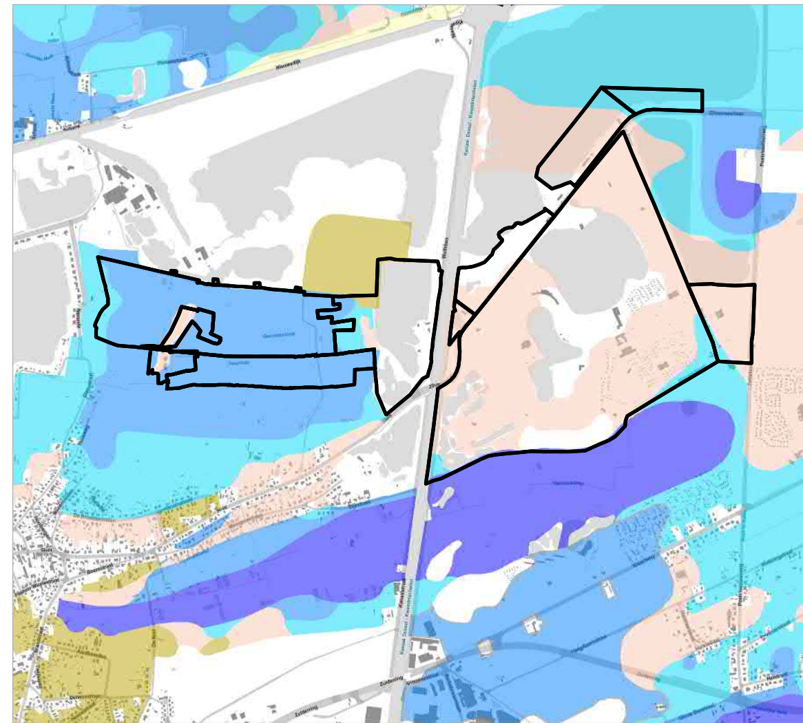
Figuur 2.1b: Bodemkaart Schansheide en Hoofdpoort
