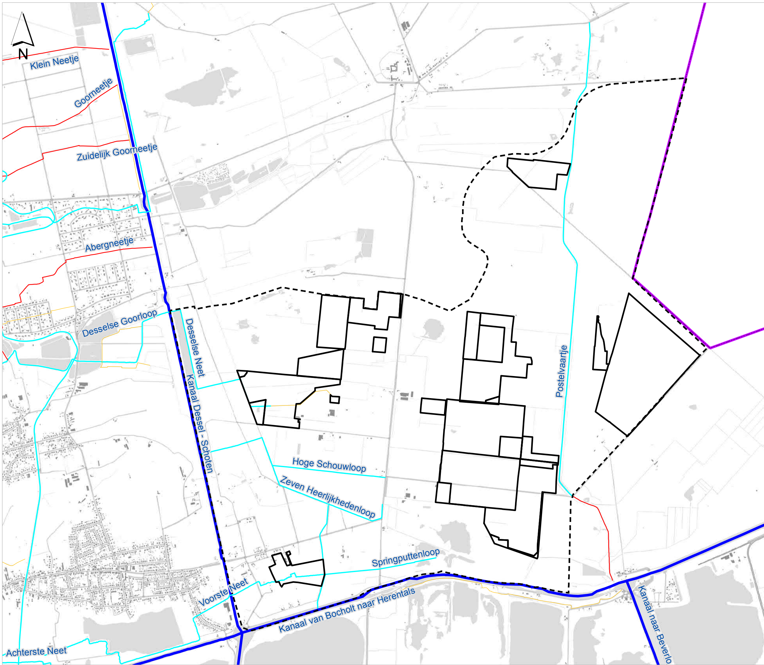
Figuur 2.2a: Waterlopen Onderzoeksruimte Mol Postel Zuid
