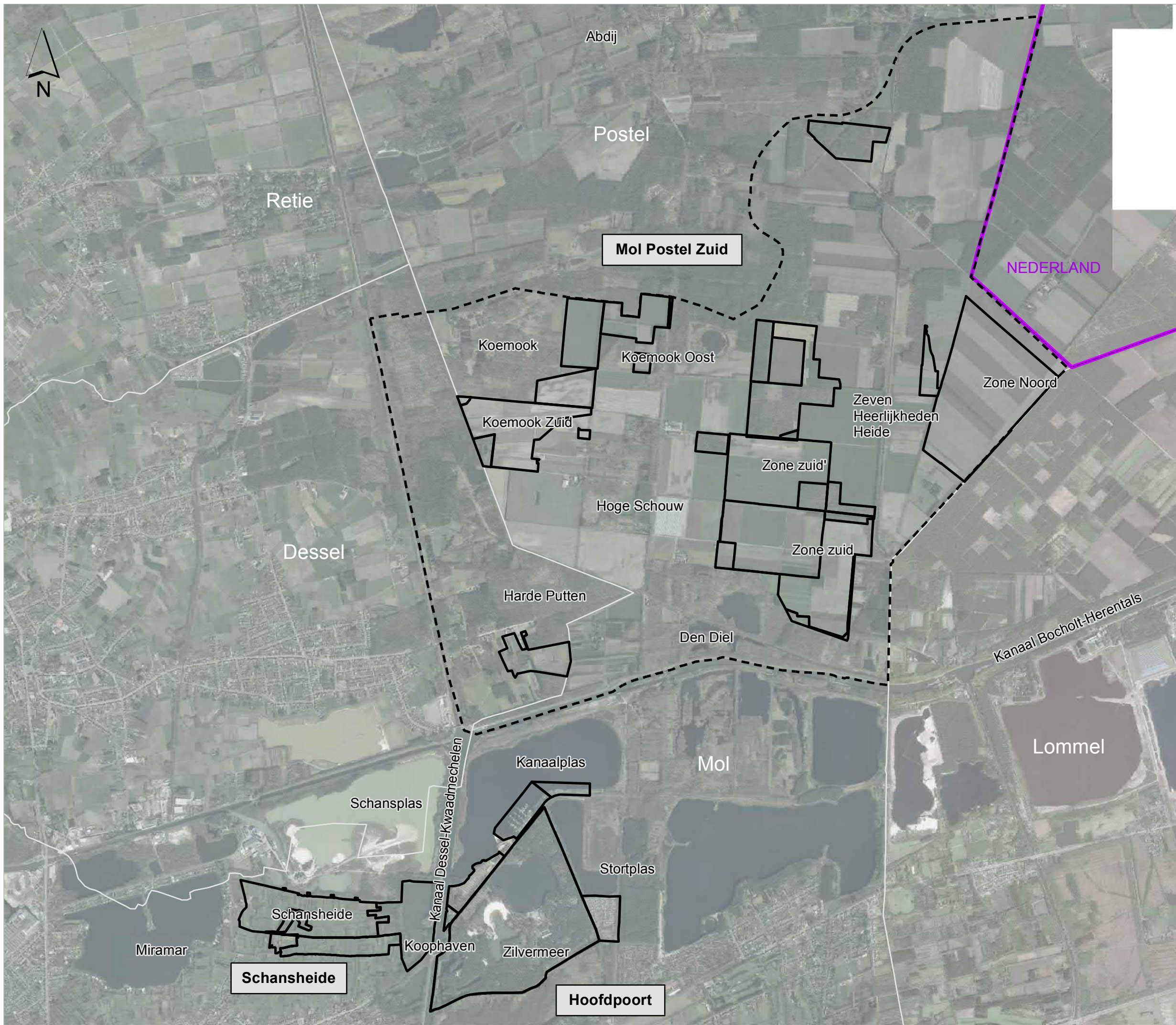
Figuur 1.1: Situering van de plangebieden en toponiemen
