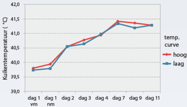
Figuur 4: Verloop van de kuikentemperatuur in het begin van de ronde bij normale/zware ééndagskuikens (leeftijd moederdieren > 38 weken / gemiddelde van 3 rondes)
