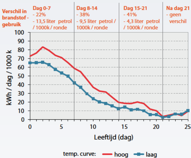
Figuur 8: Verloop van het energieverbruik voor de verwarming (gemiddelde van 6 rondes, in kWh / dag / 1000 kuikens)
